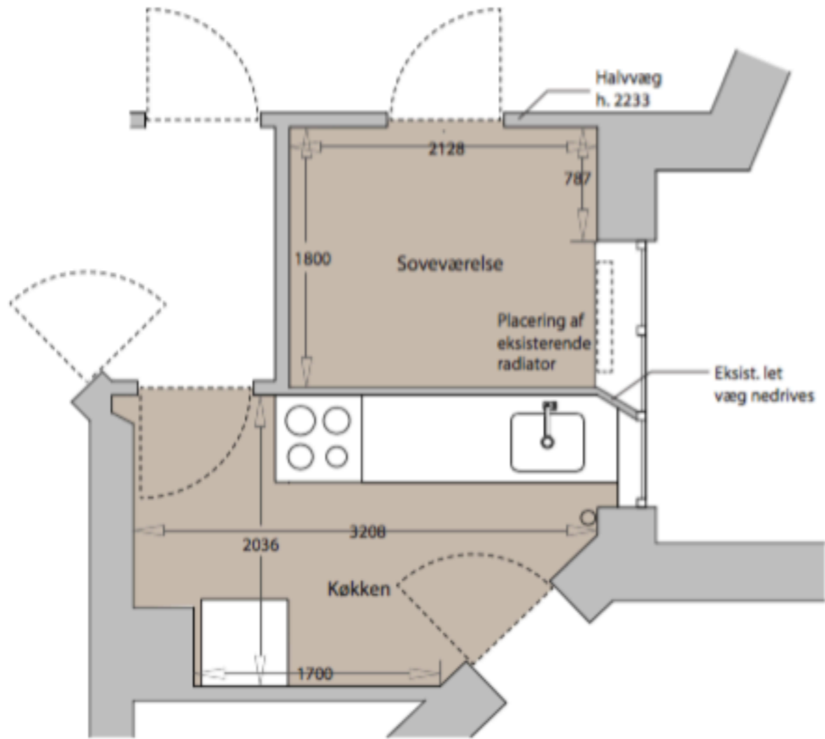
Eksisterende forhold 1:50
