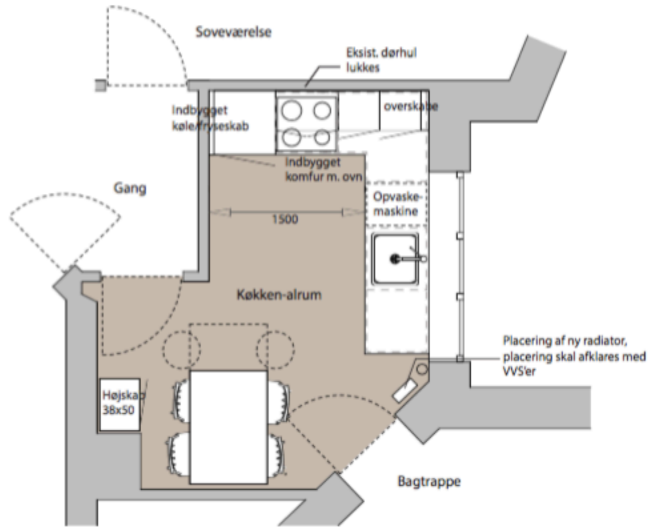
Fremtidige forhold 1:50
